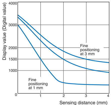
E2C-EM02H
