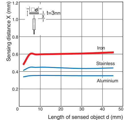
E2C-EDR6-F
