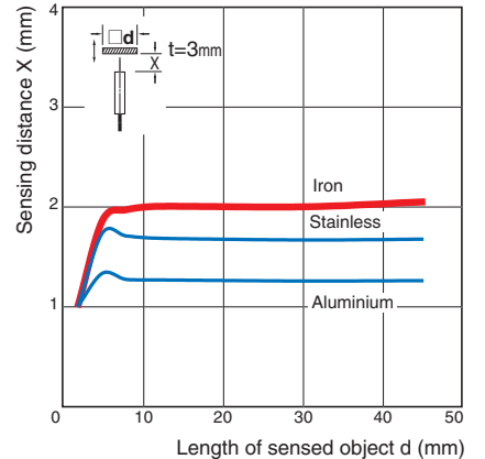
E2C-ED02(-□)/EM02(-□)
