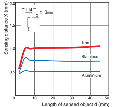
E2C-ED01(-□)
