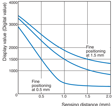
E2C-EV05(-□)
