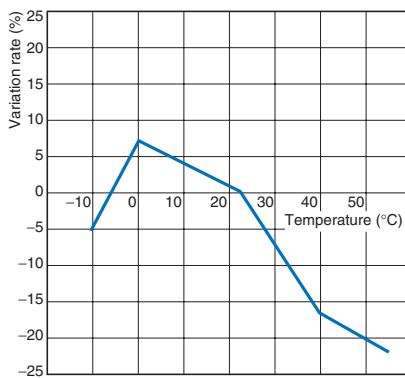
E2J-W10MA
