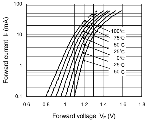
I_{FP} - V_{FP}
