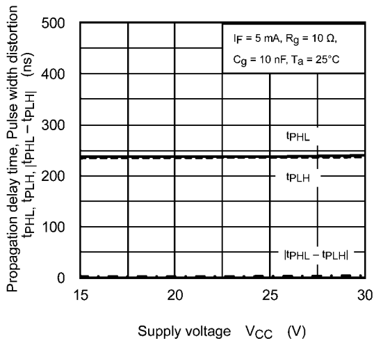
Fig. 12.2.15 t_{PHL} , t_{PLH} , |t_{PHL}-t_{PLH}| - V_{CC}
